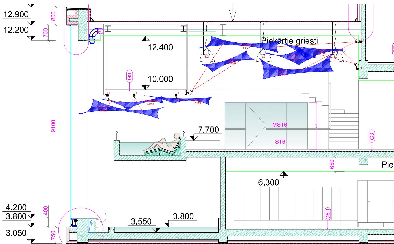
GRIEZUMS 1-1
